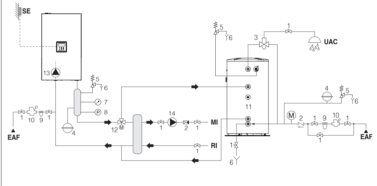
Schema 5: circuito con modulo collegato con impianto di riscaldamento e serbatoio A.C.S tramite separatore
