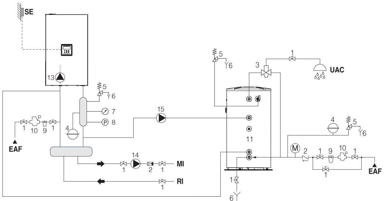
Schema 4: circuito con modulo collegato con serbatoio A.C.S. e con impianto di riscaldamento tramite separatore
