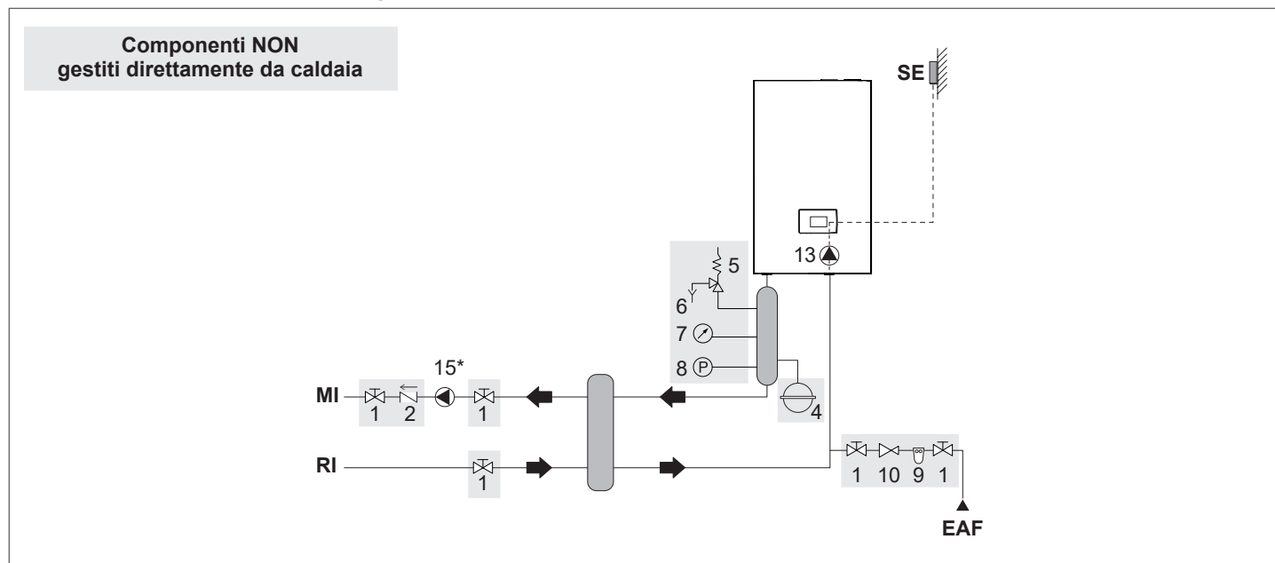
Schema 3: circuito con caldaia collegata con impianto di riscaldamento tramite separatore
