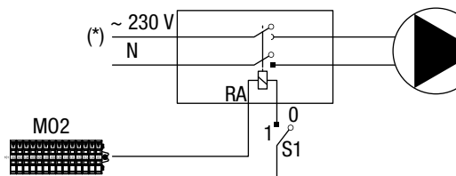
S1 - Sezionatore
