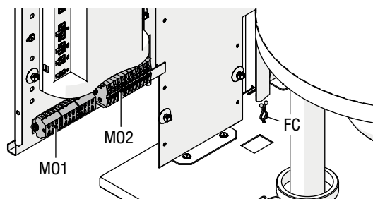
M01 - Morsetteria segnali di controllo
