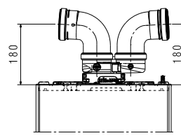
SISTEMA SDOPPIATO Ø80+80 mm CON ADATTATORE COMPATTO
