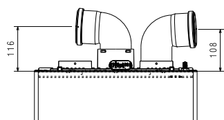
SISTEMA SDOPPIATO Ø80+80 mm
