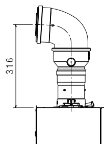
CONCENTRICO Ø80-125 mm
