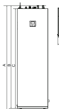
Versione L con bollitore 240-litri
