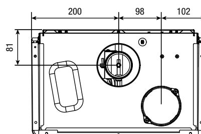
Vista dall'alto
