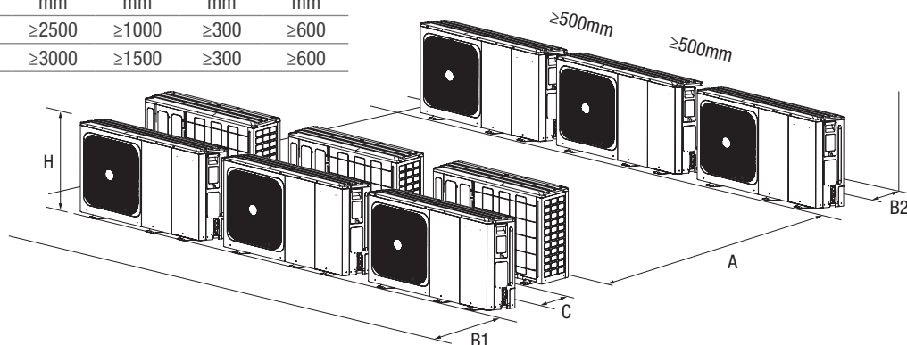
Nel caso di installazione su più file
