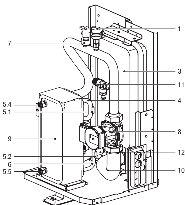
4/6 kW senza riscaldatore di backup
