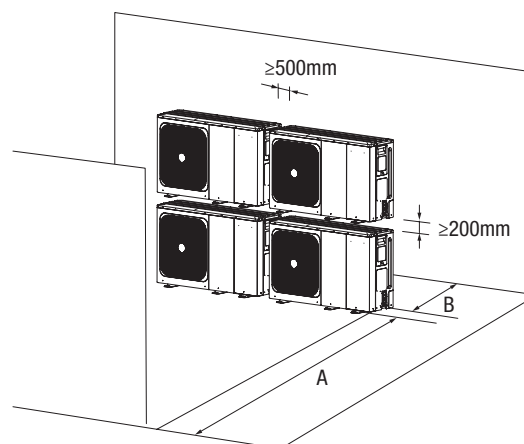
Nel caso di installazione sovrapposta
