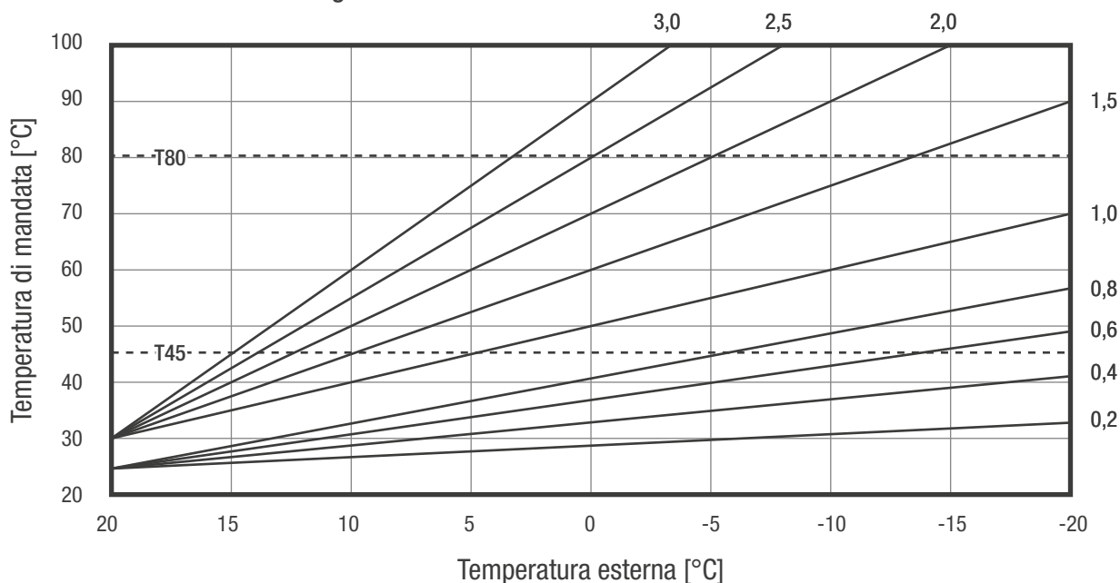
Curve di termoregolazione
