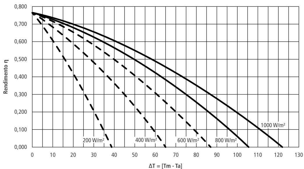
Curve di efficienza - CFS-20/4 A
