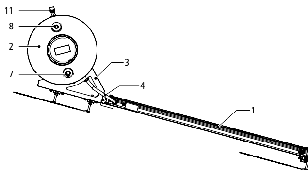
Vista laterale
