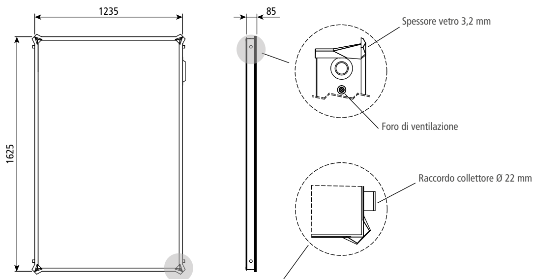
Collettore CFS-20/4 A
