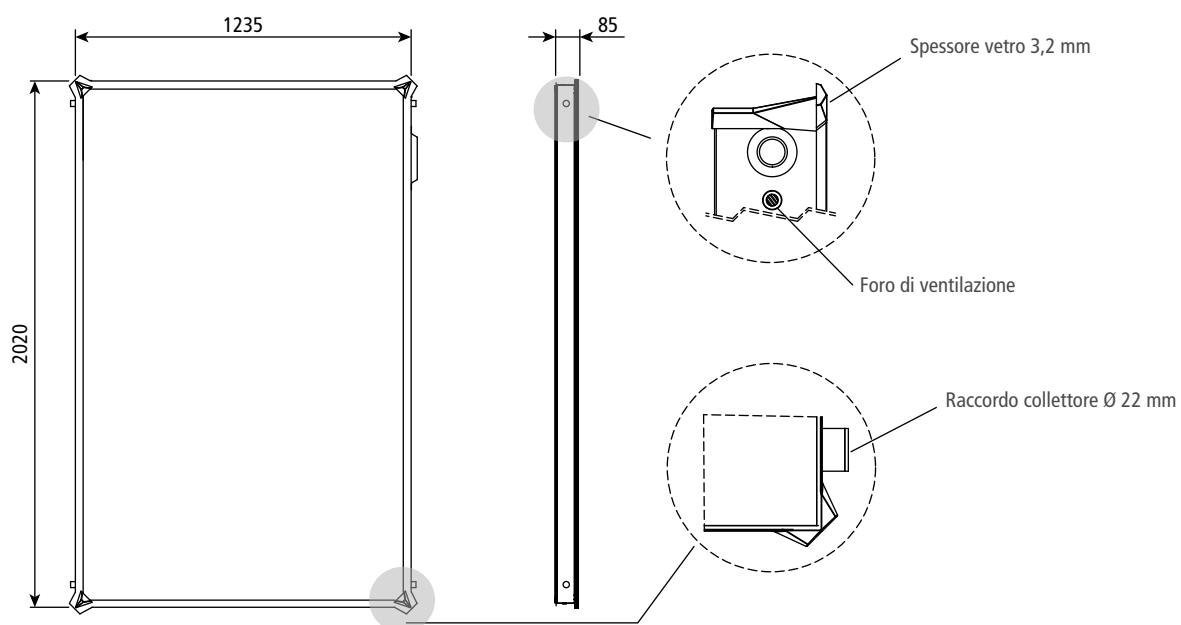
Collettore CFS-25/4 A
