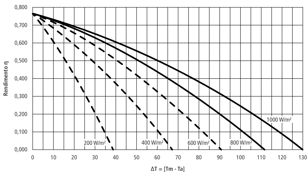
Curve di efficienza - CFS-25/4 A
