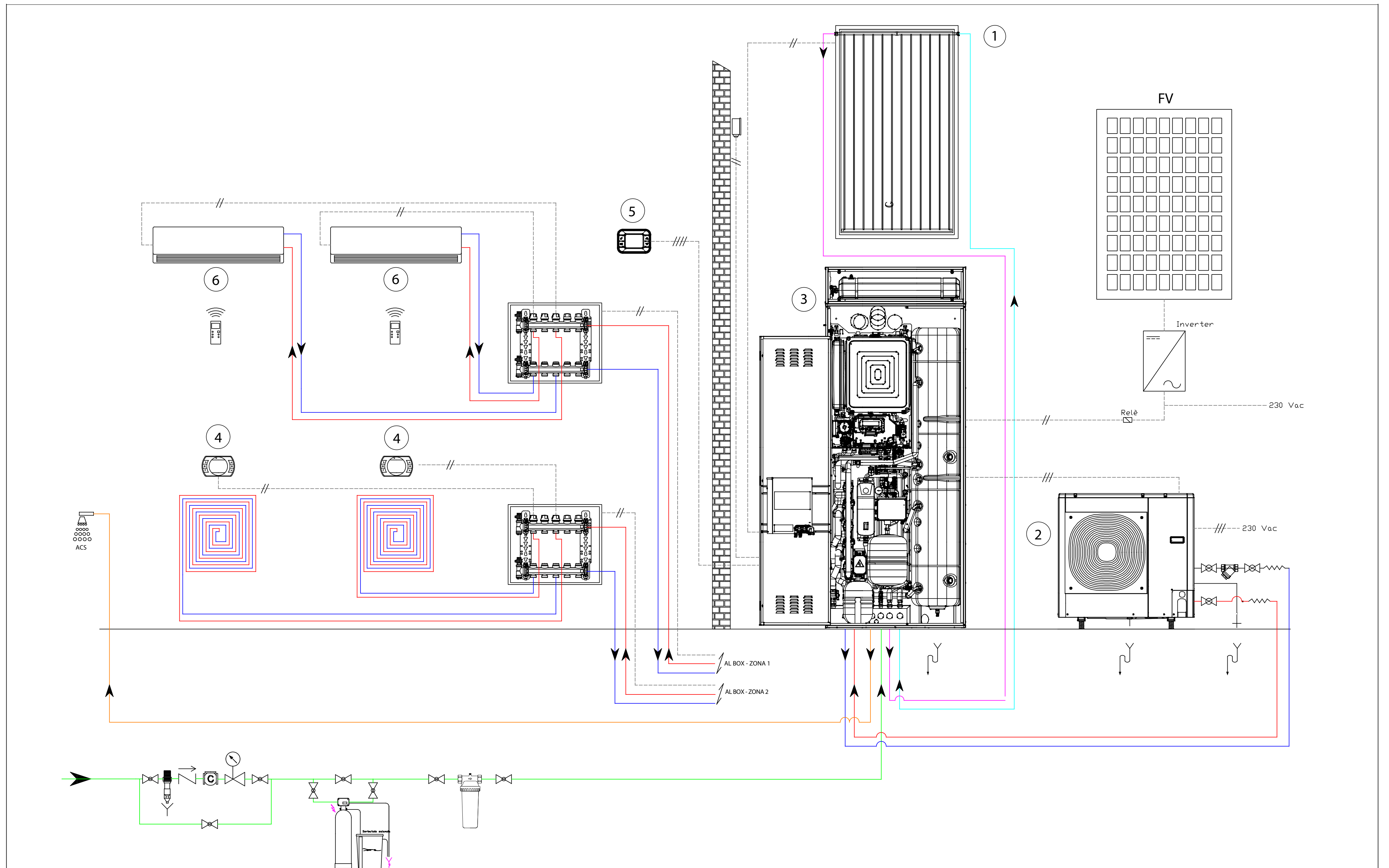
Schema di impianto puramente indicativo
