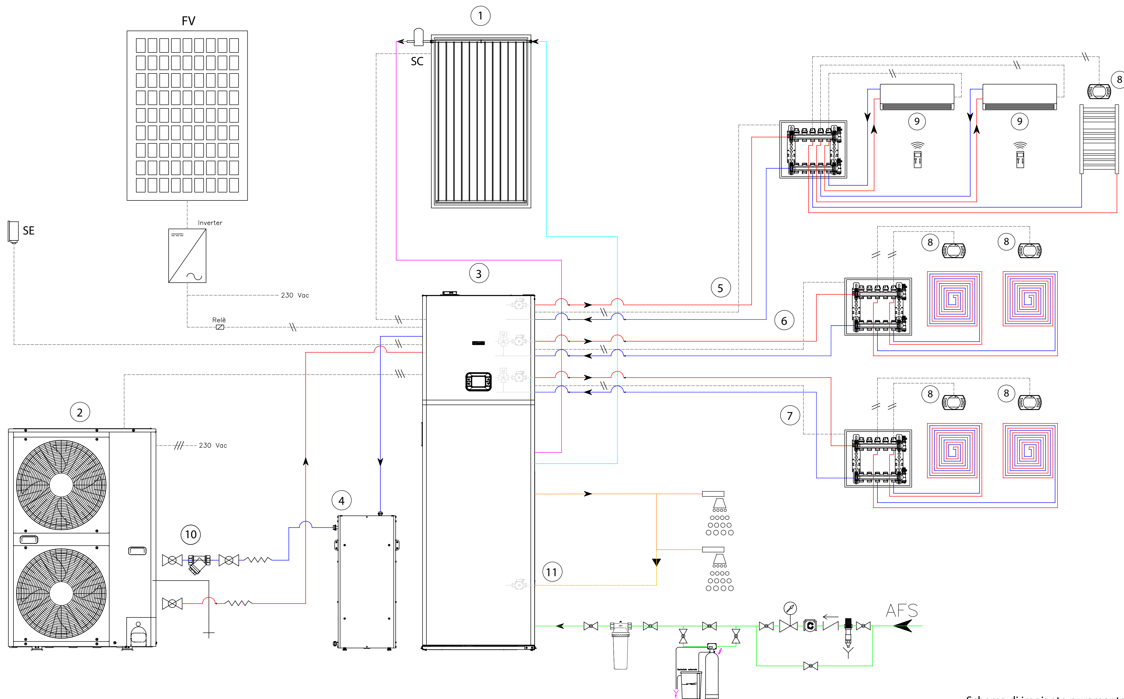
Schema di impianto puramente indicativo
