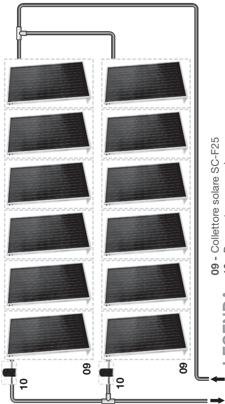
COLLEGAMENTO INVERSO PER EQUILIBRARE LE PERDITE DI CARICO NELLE BATTERIE DEL CIRCUITO - NON NECESSITA DI REGOLATORI
